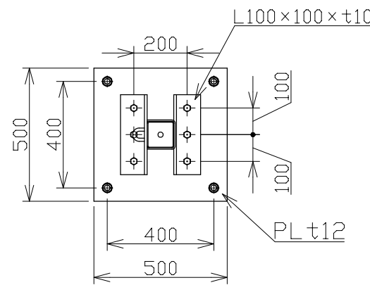
B-B'矢視図 1/20
