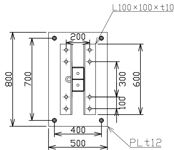
B-B'矢視図 1/20
