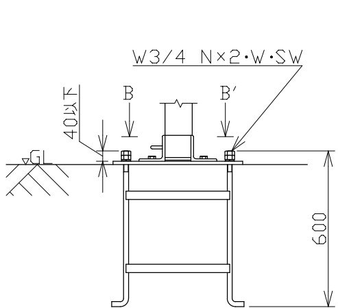
アンカーボルト詳細 1/30
