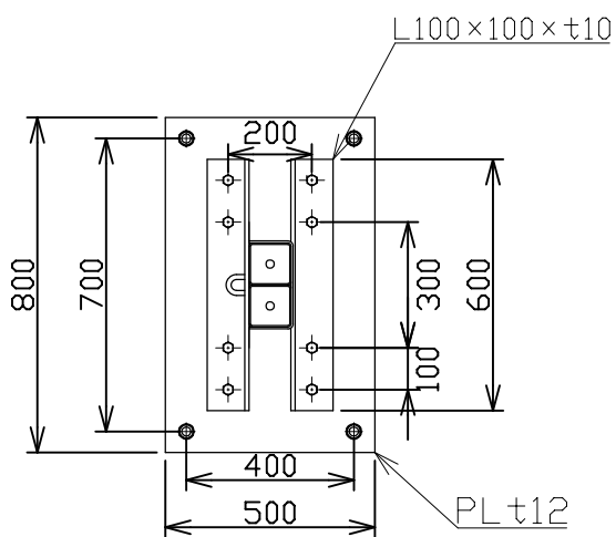
B-B'矢視図 1/20
