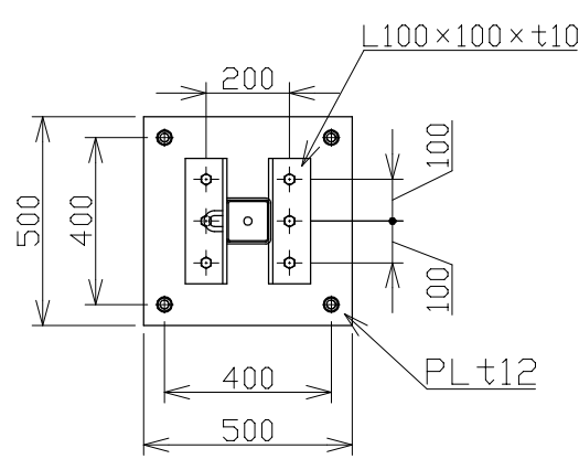
B-B'矢視図 1/20
